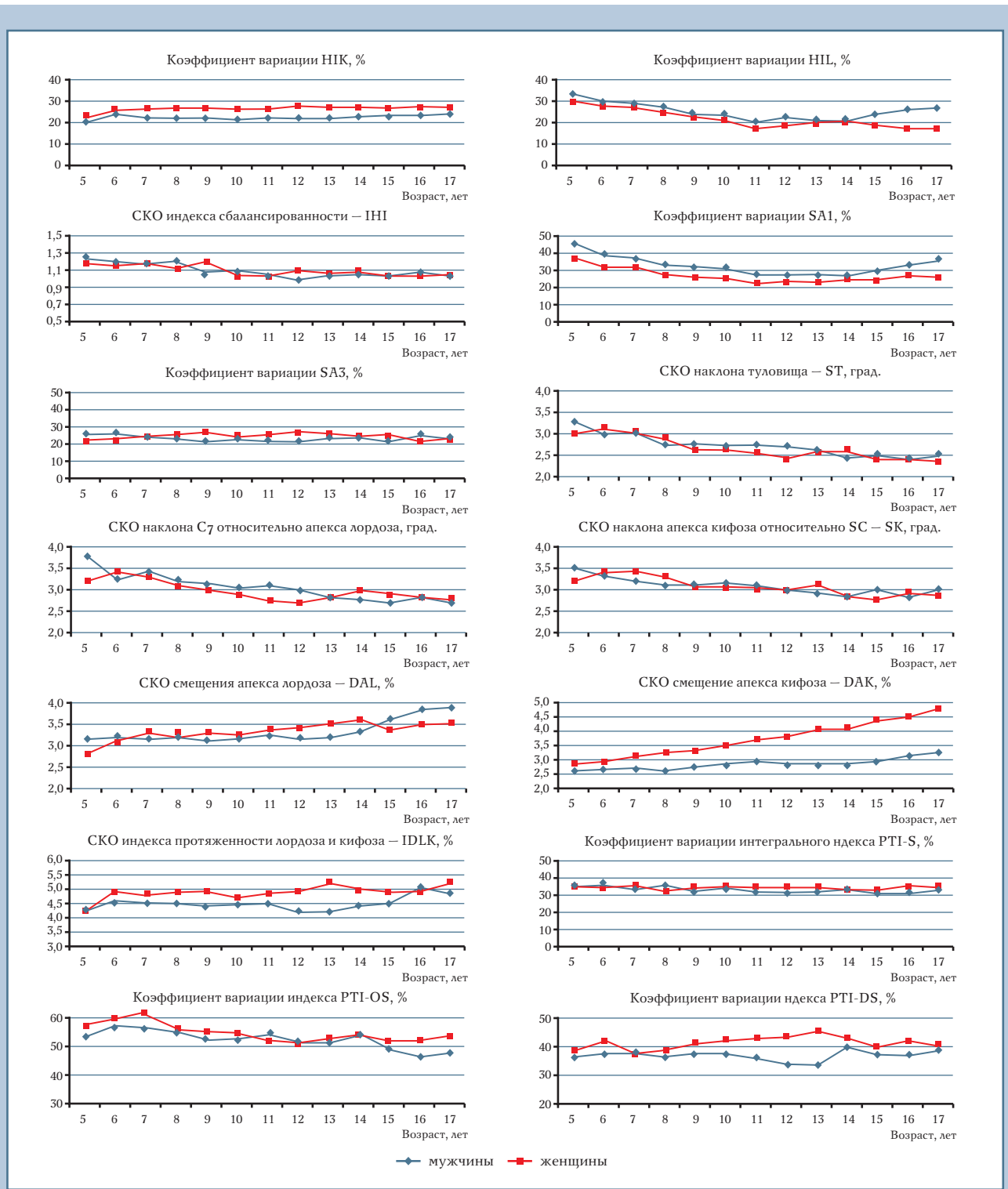
Рис. 6 Возрастная динамика коэффициента вариации и среднеквадратического отклонения топографических параметров, описывающих состояние осанки в сагиттальной плоскости
